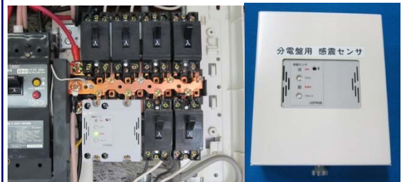
旧規格分電盤内 組込可能
